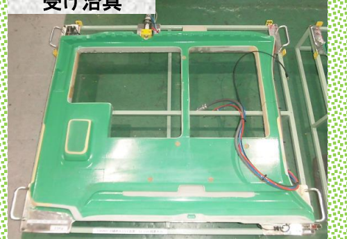
受け治具
